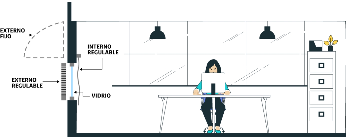
Figura 3.2.1.7. a. Ejemplo de dispositivos para controlar el ingreso de la luz diurna. (Fuente propia)
