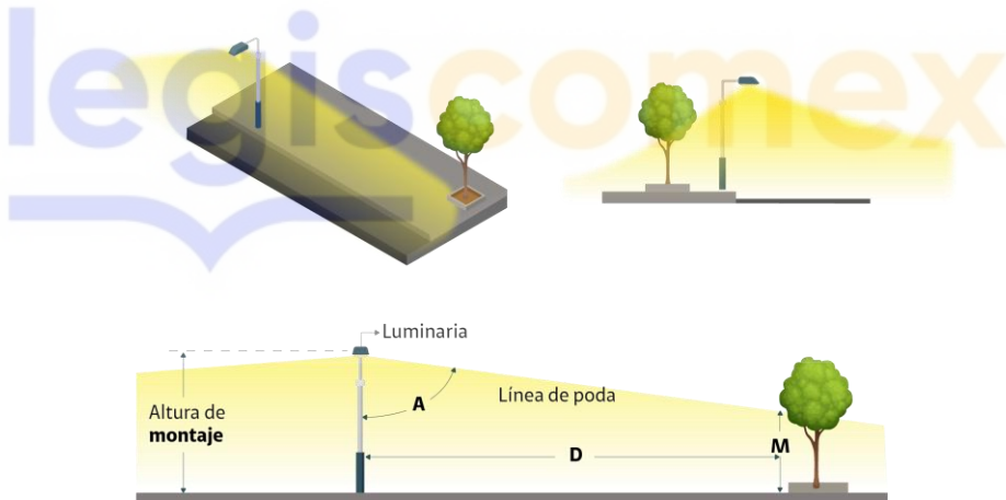
Figura 3.3.1.7. a. Separación mínima entre los árboles y los postes con las luminarias de alumbrado público, para evitar sombras sobre la vía (Fuente: Recomendaciones para la iluminación de carreteras y túneles. Gobierno de España).
