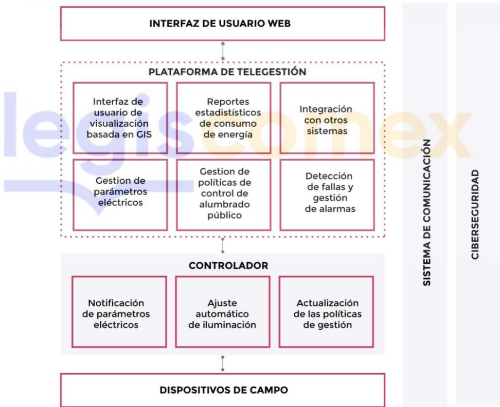
Figura 3.7.1. a Arquitectura funcional de un servicio de telegestión para alumbrado público. (Fuente propia)
